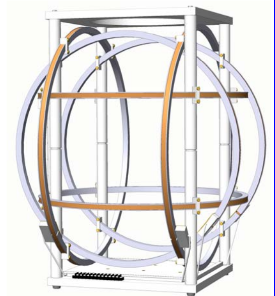
Fig. 1: BH600-3-B / 3 axes: X, Y, Z
