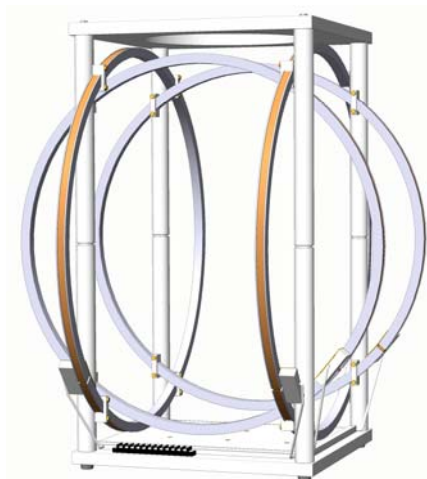
Fig. 2: BH600-2A-B / 2 axes: X, Y
